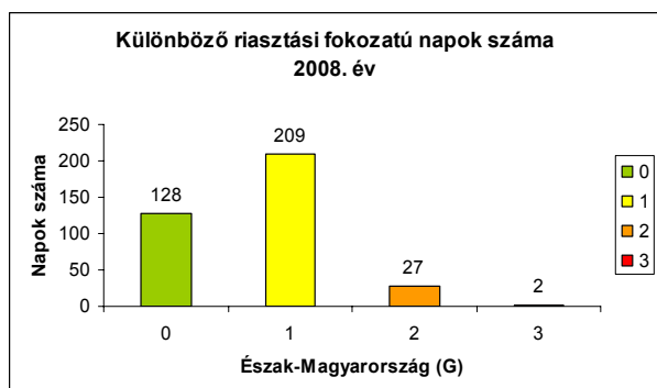
3. ábra. Az év egyes napjain kiadásra került legmagasabb szintű riasztásokat alapul véve az egyes fokozatok (zöld, sárga, narancs, piros) napjainak száma országosan (bal-felső ábra) és az egyes régiókban.
