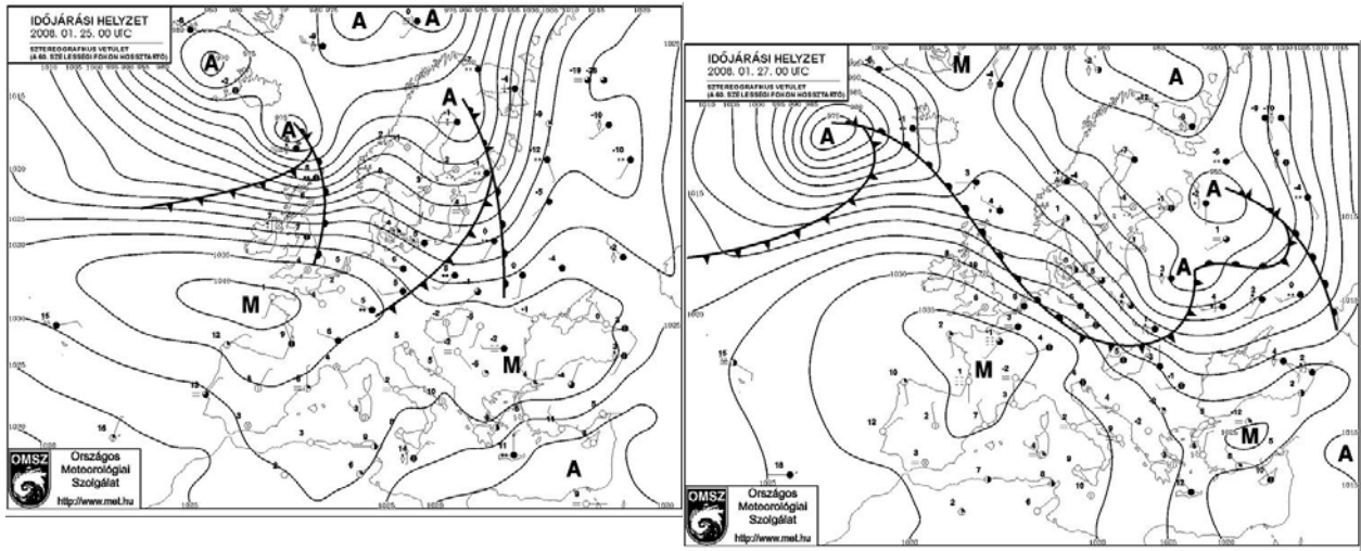
2. ábra: Szinoptikus időjárási helyzet az atlanti-európai térségben a) 2008. január 25-én 00 UTC-kor és b) 2008. január 27-én 00 UTC-kor.
