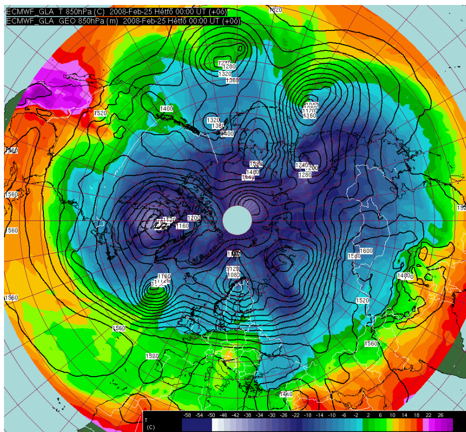
2. a) ábra : A 850 hPa magassági mezeje (folytonos vonalak) és a hőmérséklete 2008.02.25. 00 UTC-kor az ECMWF analízis alapján. A Sziklás hegység keleti oldalán látható depresszióból alakult ki az Emma.
