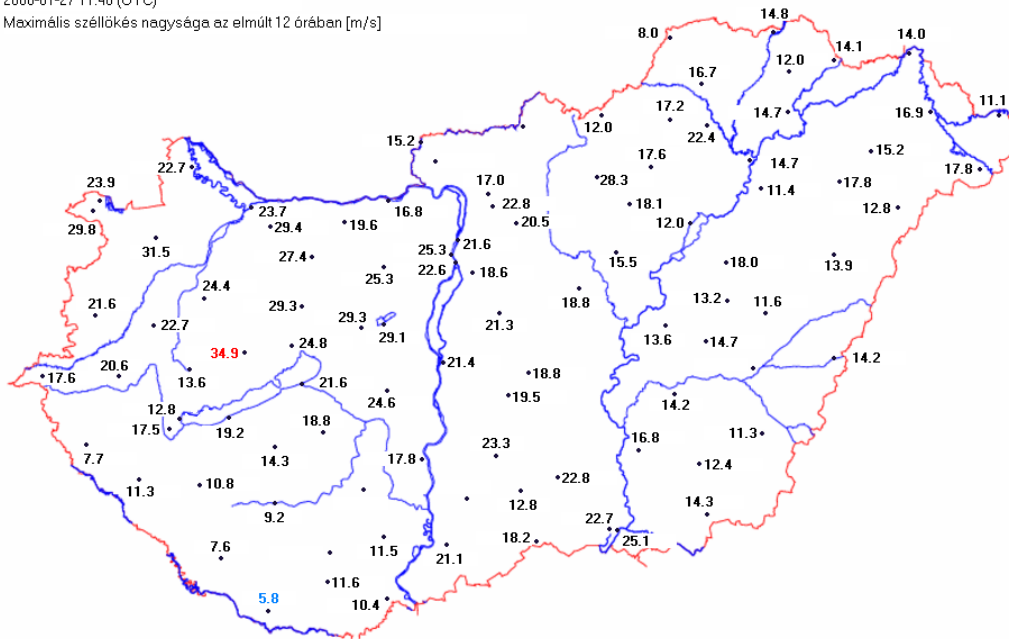
8. ábra: Maximális szélsebesség 2008. január 27-én a nap első 12 órájában
