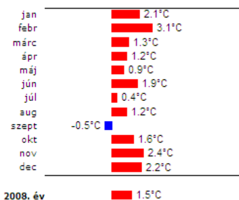
Az országos havi középhőmérséklet eltérése a sokévi (1971-2000-es) átlagtól 2008-ban (15 állomás homogenizált, interpolált adatai alapján)
