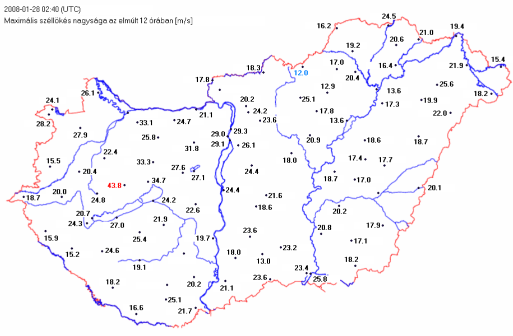
10. ábra: Maximális szellőkés nagysága 2008. január 27-e 14.40 UTC és 2008. január 28-a 02:40 UTC között.
