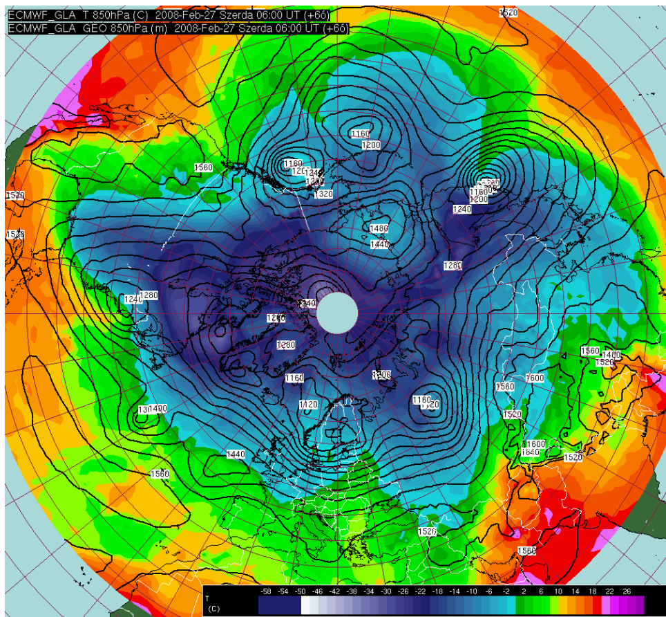
2. b) ábra: A 850 hPa magassági mezeje (folytonos vonalak) és a hőmérséklete 2008.02.27. 06 UTC-kor az ECMWF analízis alapján. A ciklon eléri az Egyesült Államok keleti partvidékét.
