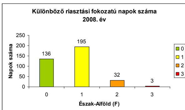
3. ábra. Az év egyes napjain kiadásra került legmagasabb szintű riasztásokat alapul véve az egyes fokozatok (zöld, sárga, narancs, piros) napjainak száma országosan (bal-felső ábra) és az egyes régiókban.
