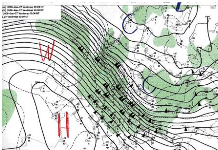
3. ábra: 500 hPa-os magassági térkép 2008.01.27. 00 UTC-kor (Az 500 hPa-os geopotenciál értéket fekete izovonalak, a hőmérsékletet szaggatott kék izovonalak, a szelet szélzászlók jelölik. A szélzászló esetében egy háromszög 25 m/s, egy hosszú vonal 5 m/s szélsőséget jelent.)
