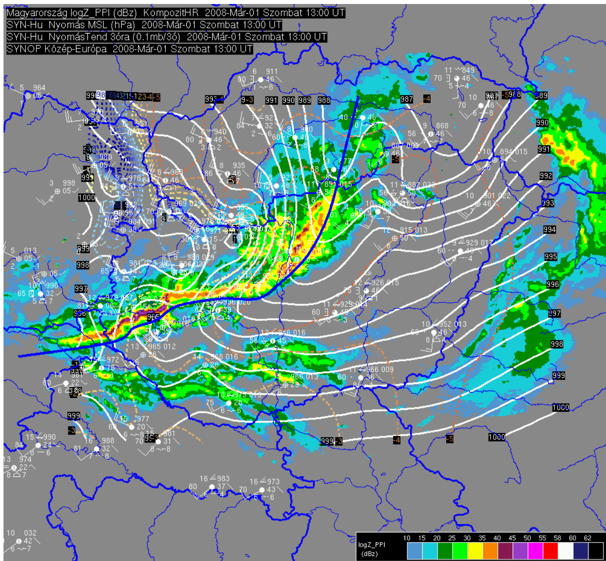
6. b) ábra: Országos, kompozit radarkép, a tengerszintű légnemű és a felszíni mérések 2008.03.01. 13 UTC-kor. A front elhelyezkedését folytonos kék vonallal jelöltük.
