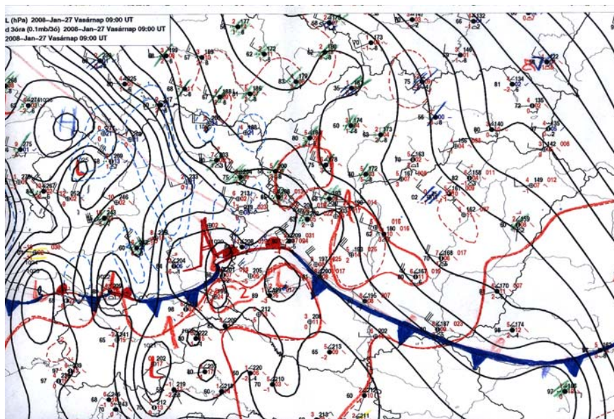
6. ábra: 09 UTC-s helyzetkép a Kárpát-medencében 2008. január 27-én
