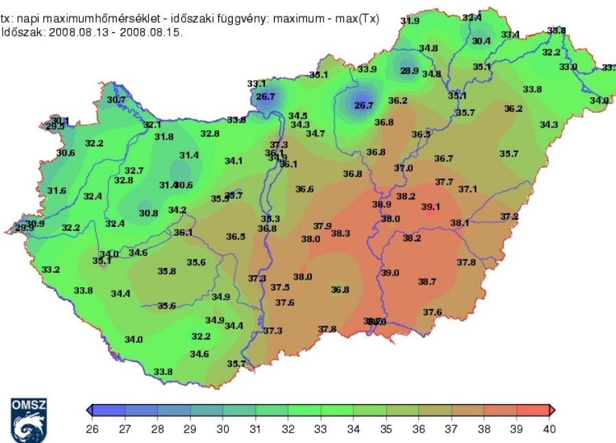
12. ábra: Legmagasabb mért hőmérsékletek augusztus 13. és 15. között. Az időszak, és egyben az év legmagasabb hőmérsékletét Turkevényen mérték augusztus 15-én, 39,1 °C fokat.
