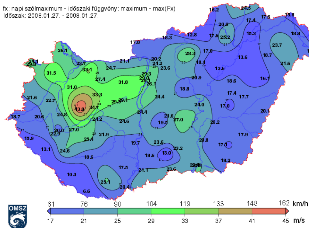
11. ábra: 2008. január 27-én előfordult legerősebb szélökések
