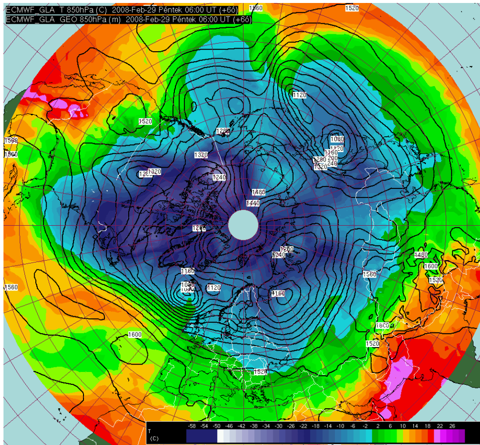
2. d) ábra: A 850 hPa magassági mezeje (folytonos vonalak) és a hőmérséklete 2008.02.29. 06 UTC-kor az ECMWF analízis alapján. Az Atlanti-óceán fölött felgyorsult ciklon eléri megközelíti a Brit-szigeteket.
