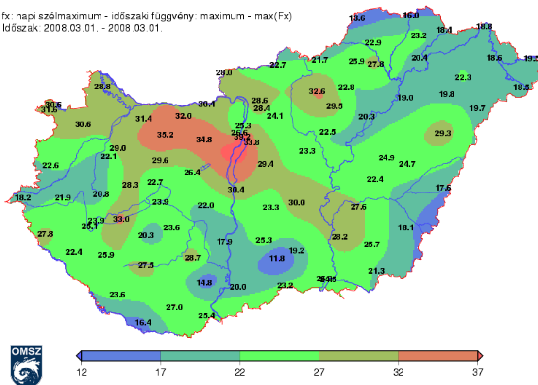
1. ábra: Magyarországon mért legerősebb szellökések 2008-03-01-én. (25 m/s \approx 90 km/h fölött erős viharról, 33 m/s \approx 120 km/h fölött orkán erejű szélről beszélünk)
