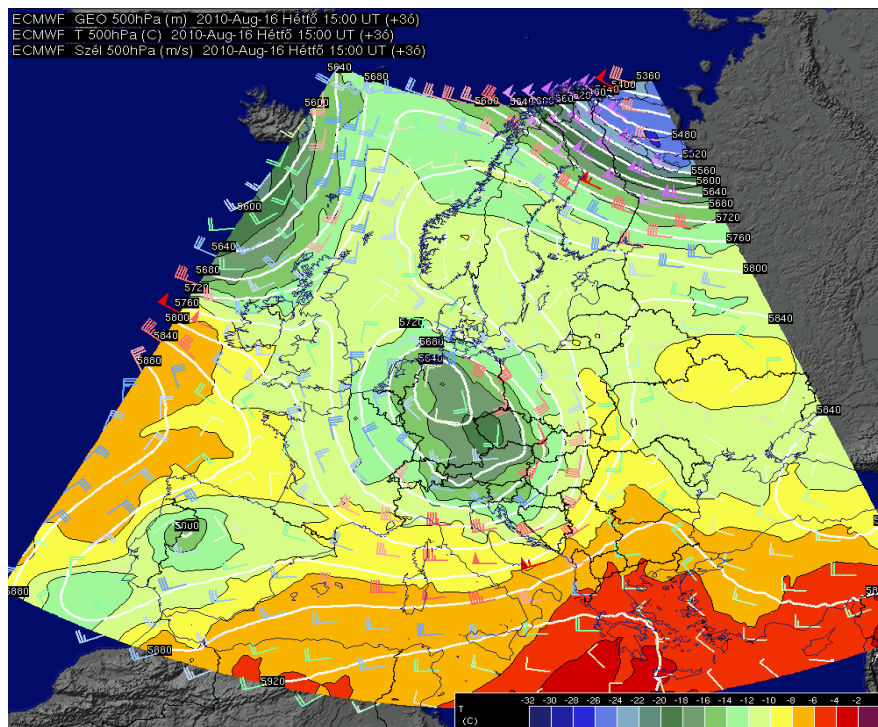
2. ábra: Az örvény elhelyezkedése 500 hPa-on 15 UTC-kor 2010. 08. 16-án. Kb. 2-3 fokos hideg advekcio ment végbe középszinteken napközben. A teknő előoldalán jelentős volt a magassági szél
