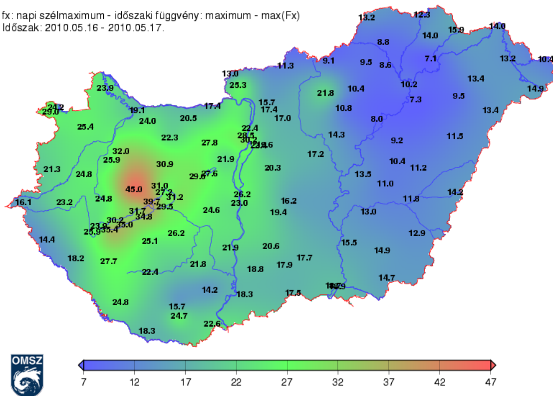
3. ábra: Maximális szellőkések 2010-05-16-17-én m/s-ban (1 m/s=3.6 km/h)
