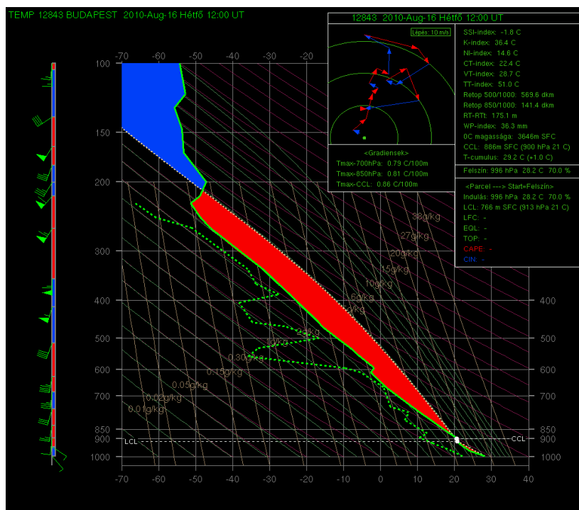
8. ábra: A budapesti rádiószondás mérés alapján a felszínalapi CAPE értéke 3000 J/kg felett volt Budapesten, megfelelően nedves profil mellett. Ez az érték az USA-ban is megállná a helyét.
