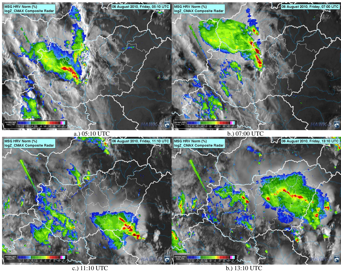
4. ábra: Szimultán műholdkép és radarkép 05, 07, 11 és 13 UTC időpontban. A Dunántúlon kialakult éjszakai, reggeli zivatarok gyengülése után napközben Szerbia-Románia felől a korábbiaknál hevesebb zivatarok alakulnak ki és vesznek fel vonalas rendeződést az Alföldön.
