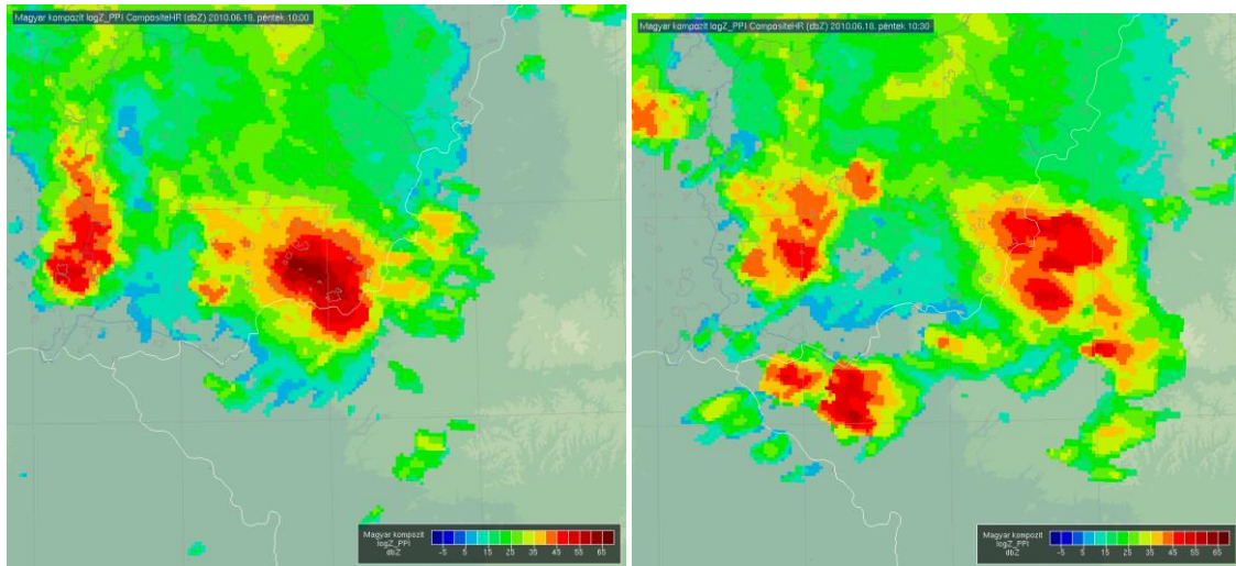
7. ábra: A zivatarrendszer átvonulása Dél-Magyarországon a radarmegfigyelések alapján.
