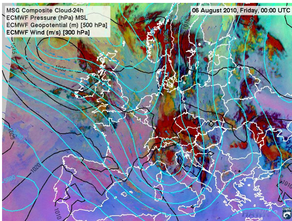
1. ábra: Tengerszintű légnyomás/fekete/, 500 hPa-os geopotenciál /türkíz/ mezeje Európa térségében 2010.08.06. 00 UTC időpontban. Az Észak-Olaszország fölötti centrummal elhelyezkedő időjárási rendszer fokozatosan kelet felé helyeződik át.
