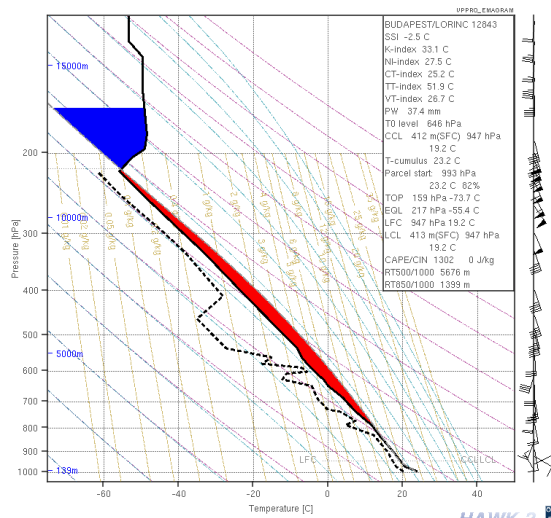
2. ábra: Budapesti rádiószondás felszállás augusztus 6-án 00 és 12 UTC időpontban. A déli órákra a jelentős labilitás mellett az alsó 3 km-ben a szélnyírás is igen kedvezően alakult szervezett konvekció kialakulásához (talajközben gyenge keleti szél, 3-4 km-en már 15-20 m/s déli, délnyugati szél figyelhető meg.)
