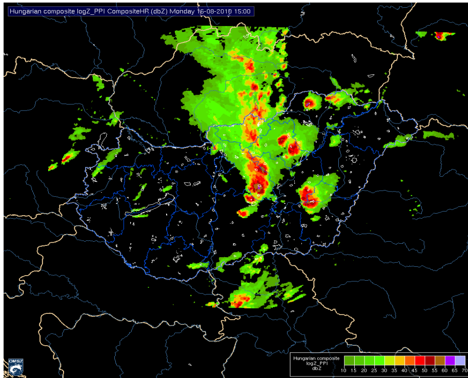
7. ábra: A zivatarrendszer elhelyezkedése 15 UTC-kor. A vonal előtt egyedi heves szupercellás zivatarok pattannak ki, amelyek a heves események egész arzenálját vonultatták fel
