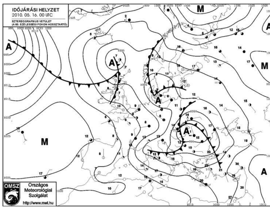
1. ábra: Az európai időjárás helyzet 2010.05.16. 00 UTC-kor
