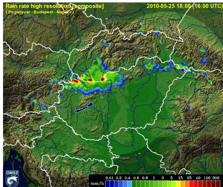
4. ábra: Országos radarkép 2010. május 25. 16:00 UTC
