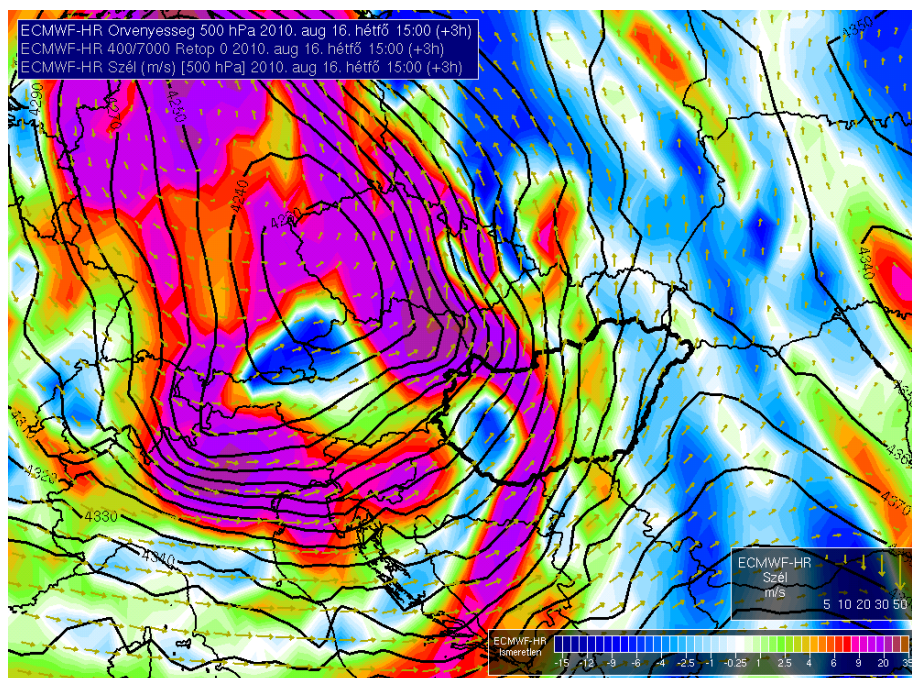
6. ábra: Vonalas kényszerhatás érkezése 500 hPa-on 15 UTC-kor
