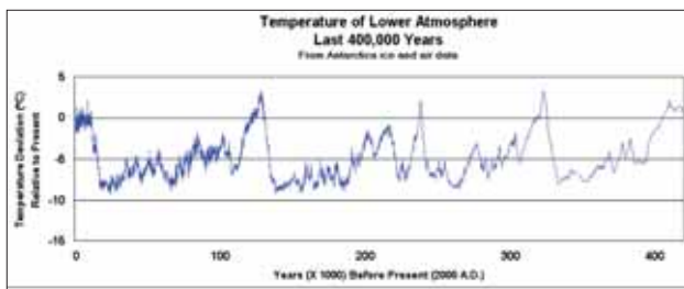
1. ábra: Az elmúlt 400 ezer év hőmérsékleti adatsora
