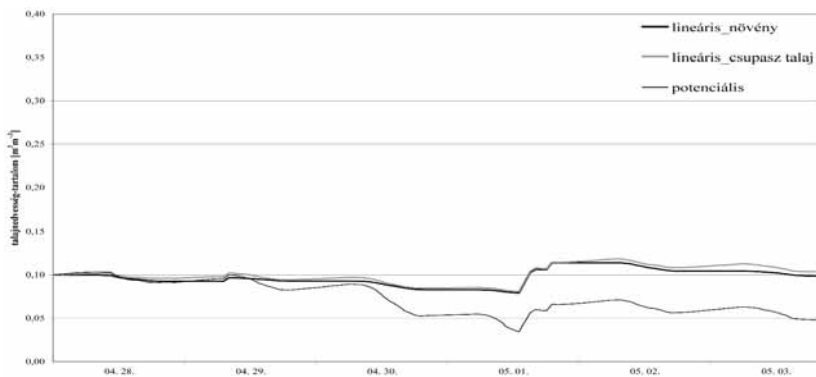
9. ábra: A csupasz talaj és a növényzet alatti talaj nedvesség-tartalmának időbeli változása (homok, lineáris forma)
