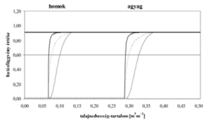
3. ábra: A növényzet párolgását jellemző \beta^v_i függvény változása a talajnedvesség-tartalom függvényében (a globálsugárzás értéke minden esetben 800 \text{ Wm}^{-2} , a szélesebbesség 2 \text{ ms}^{-1} , a levegő telített, a léghőmérséklet 25 \text{ }^\circ\text{C} )
